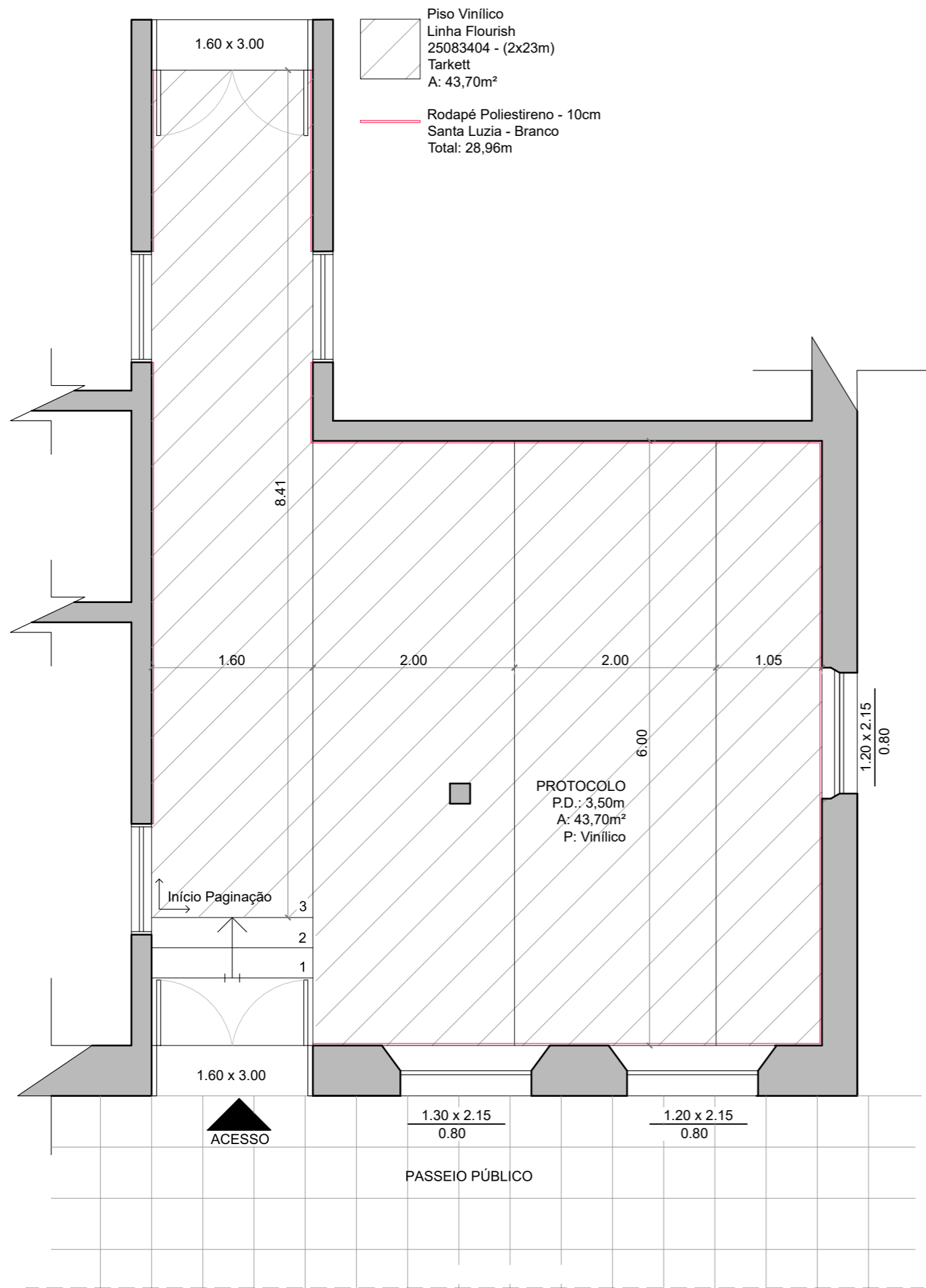
PLANTA DE PISO ESC.: 1/50
